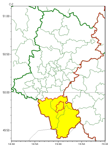
Oblodzenie 2023-11-19 04:17
